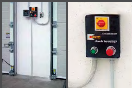
CANALINA GENERICA COPRICAVI CON QUADRO ELETTRICO CABLE CASING WITH CONTROL PANEL
