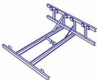
Telaio Autoportante Tassellato Per Automezzi Senza Sponda Idraulica
