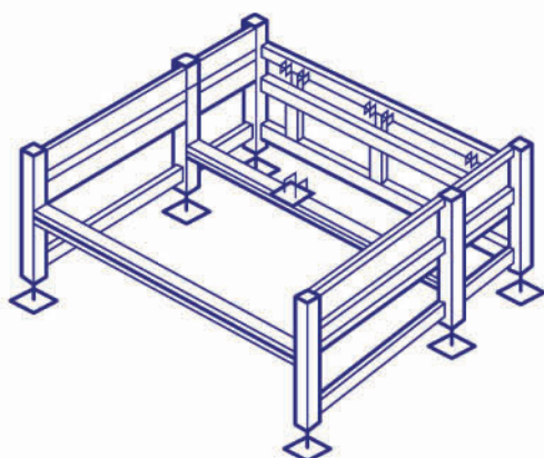
Telaio Esterno Rampa Per Automezzi Senza Sponda Idraulica
